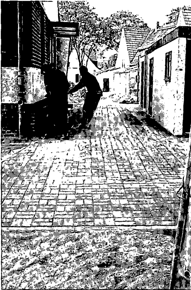
Abbildung 9: Pflaster einer Einfahrt abrütteln (Rüttelplatte mit Gummimatte) (C1 13)
