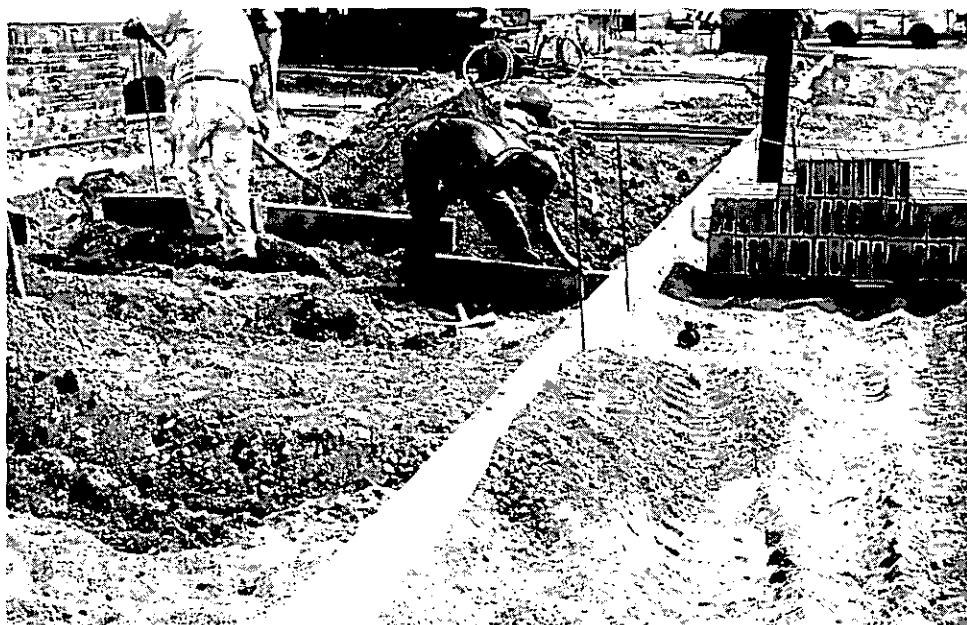
Abbildung 11: Randsteine setzen (C1 16)
